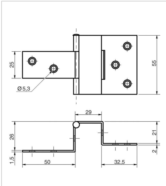
Charnière universelle acier contre coudée 270°.
