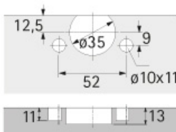
Cotes de perçage TX33/52x9 Selekt Pro 2000
