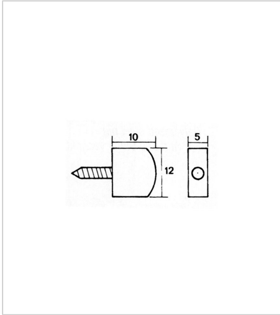
Taquet laiton avec vis double filet acier.
